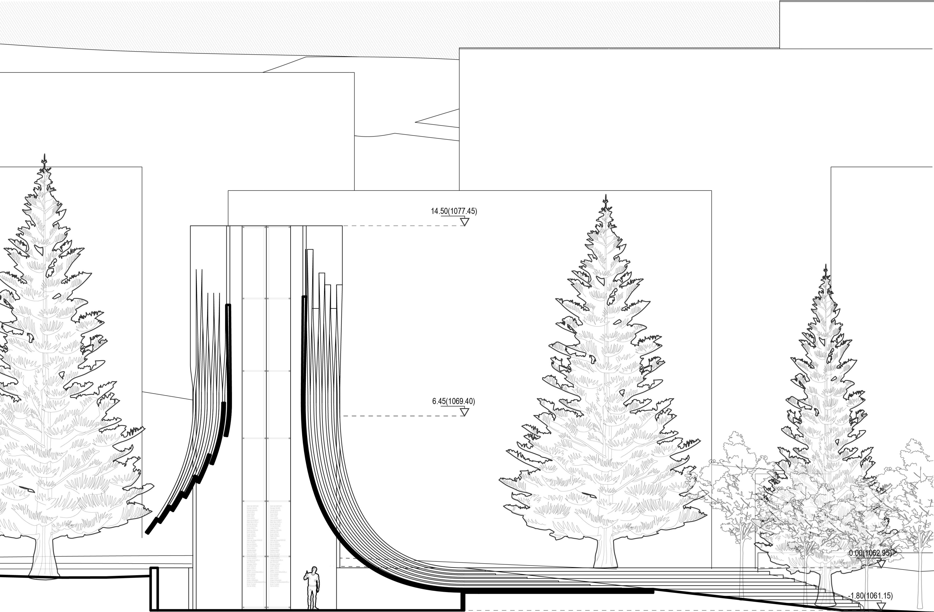
AA KESİTİ (1/100)
